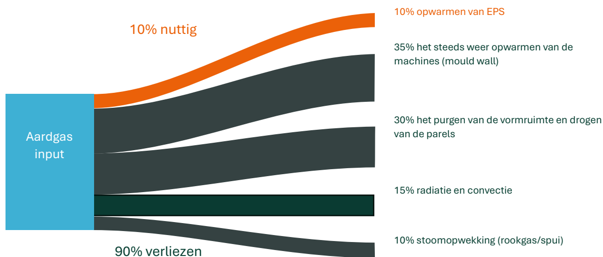
Figuur 18 - Sankey diagram thermische energie voor EPS-productie
