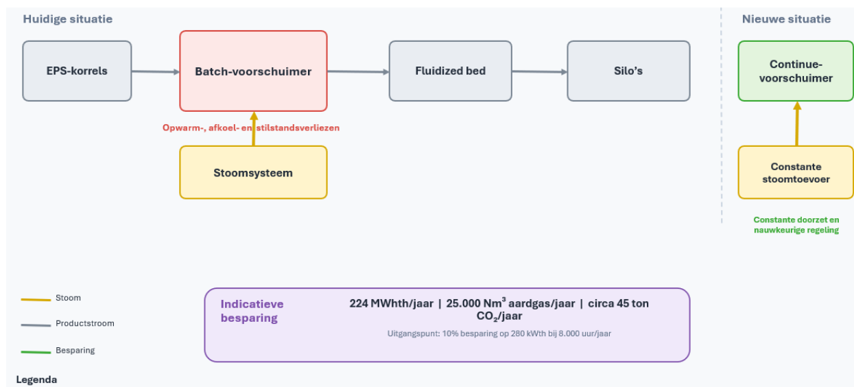
Figuur 25 – Schema maatregel 5 EPS
