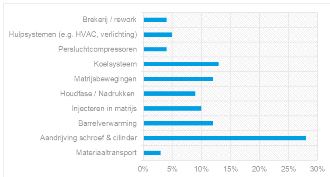
Figuur 10 - Elektriciteitsbalans spuitgietproces
