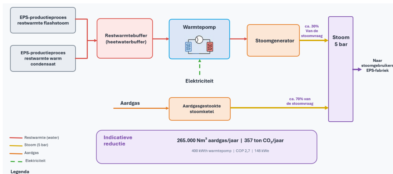
Figuur 21 – Schema van maatregel 1 EPS
