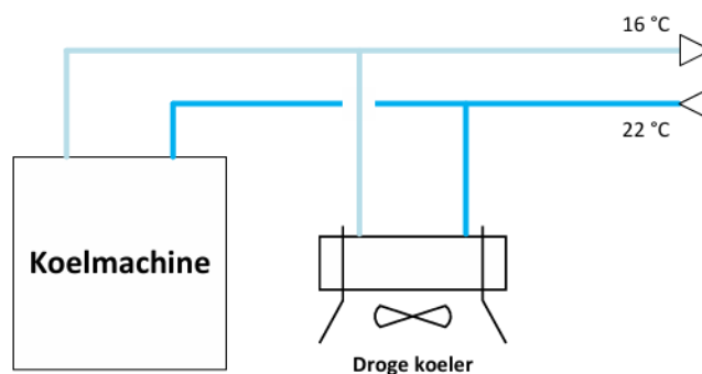
Figuur 7 - Koelsysteem incl. droge koeler
