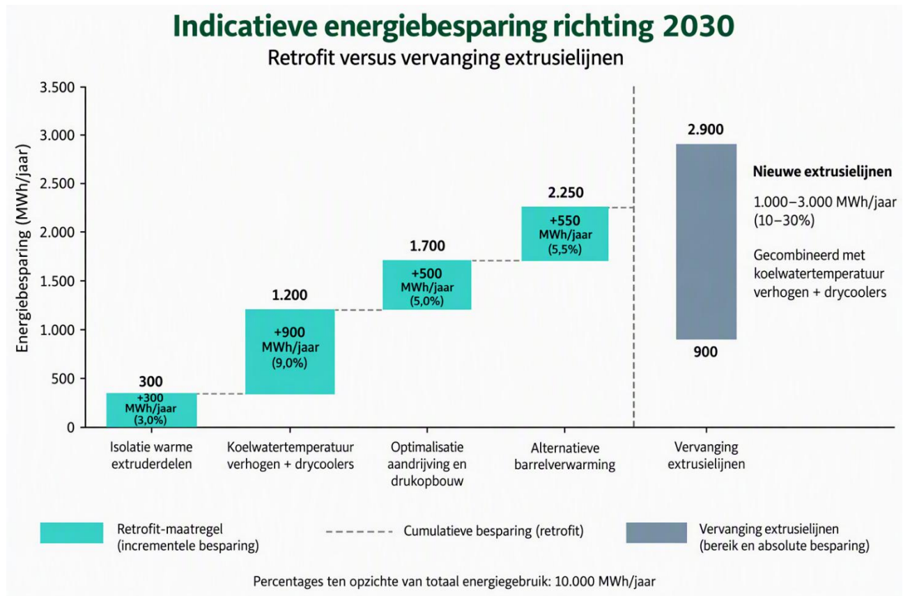
Figuur 8 – Routekaart implementatie top 5 extrusie
