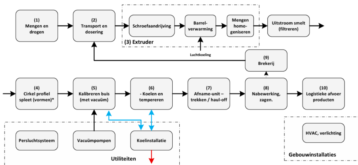
Figuur 1 – Extrusie blokschema
