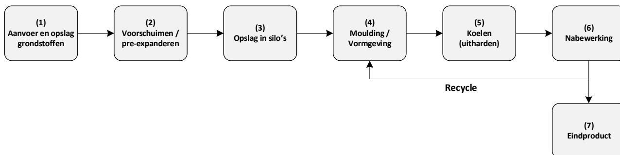
Figuur 17 – Schematische weergave productieproces EPS-producten
