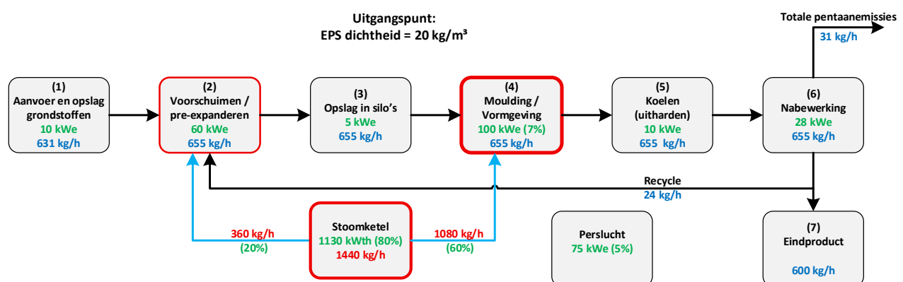
Figuur 20 – Energie- en massabalans EPS-productieproces
