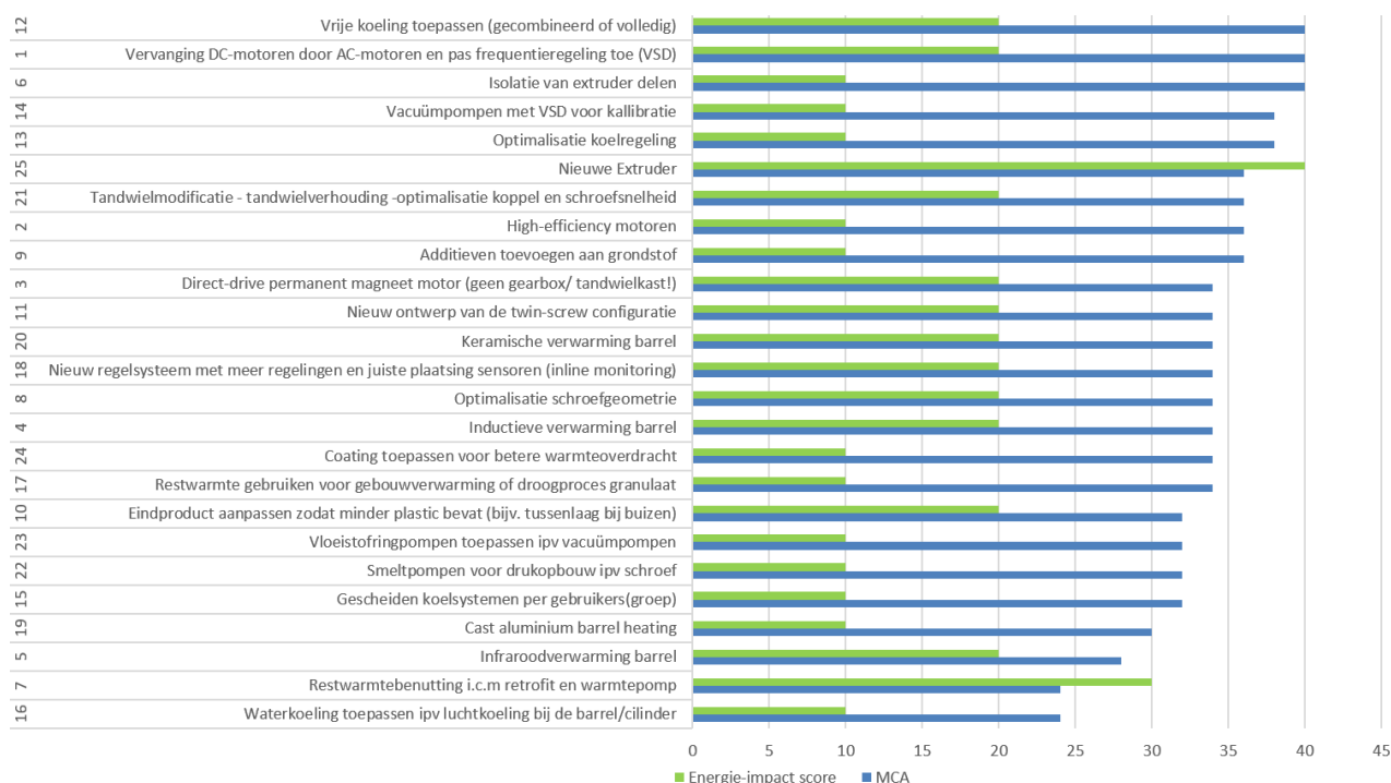
Figuur 5 - Scoring maatregelen extrusie
