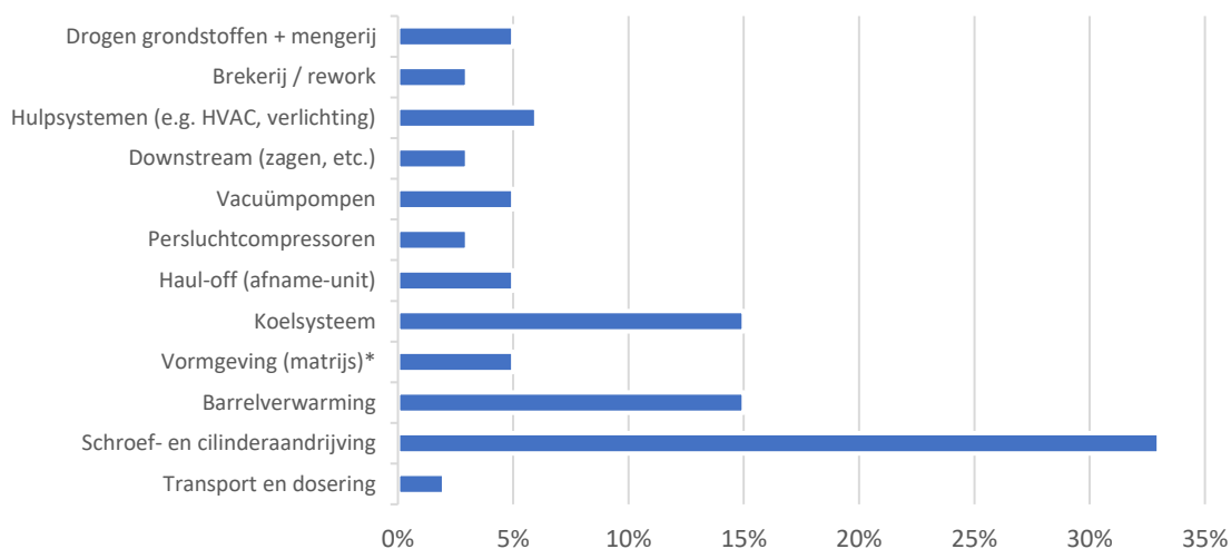
Figuur 2 – Onderverdeling elektriciteitsgebruik extrusieproces
