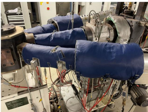
Figuur 6 - Voorbeeld van isolatie van warme extruderdelen ( voorbeeld isolatie )
