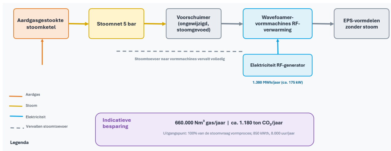
Figuur 23 – Schema voor maatregel 3 EPS
