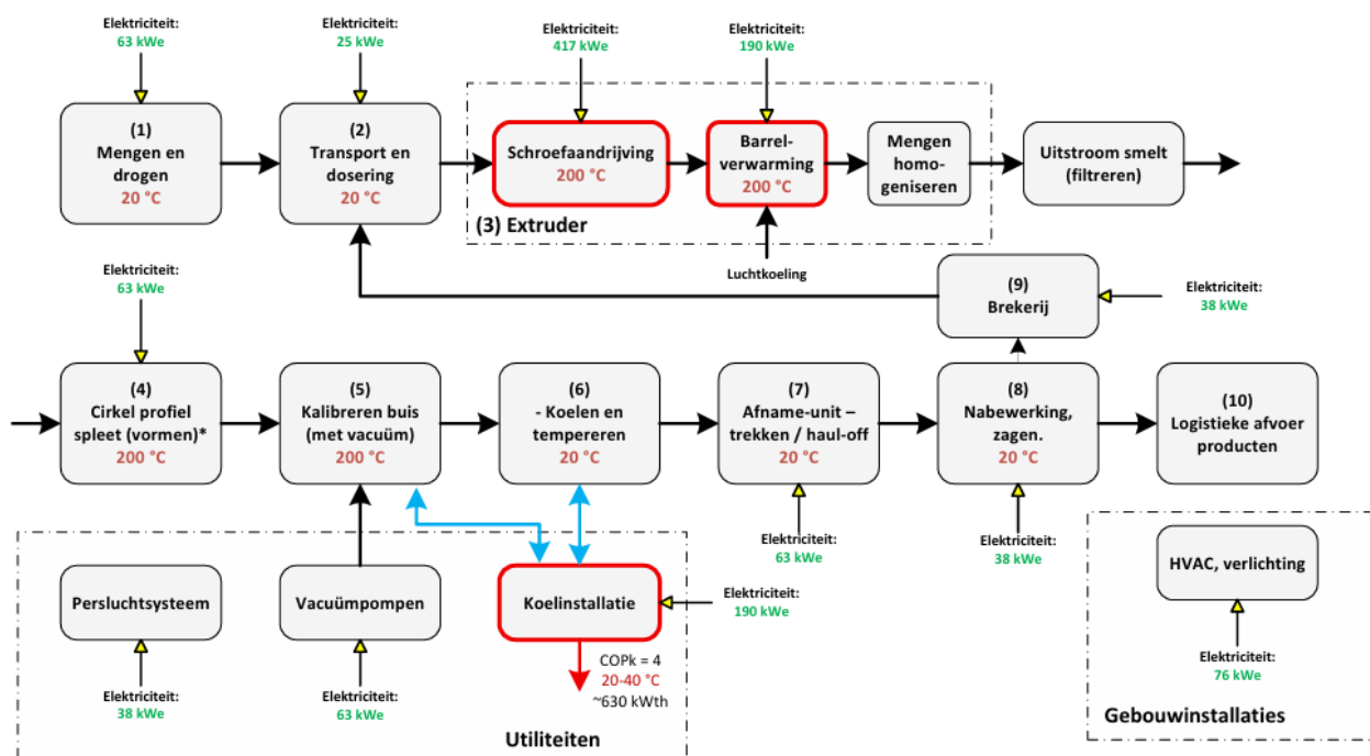
Figuur 3 – Energiebalans extrusieproces
