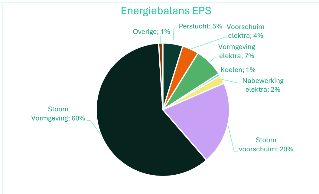
Figuur 19 - Energiebalans EPS productie
