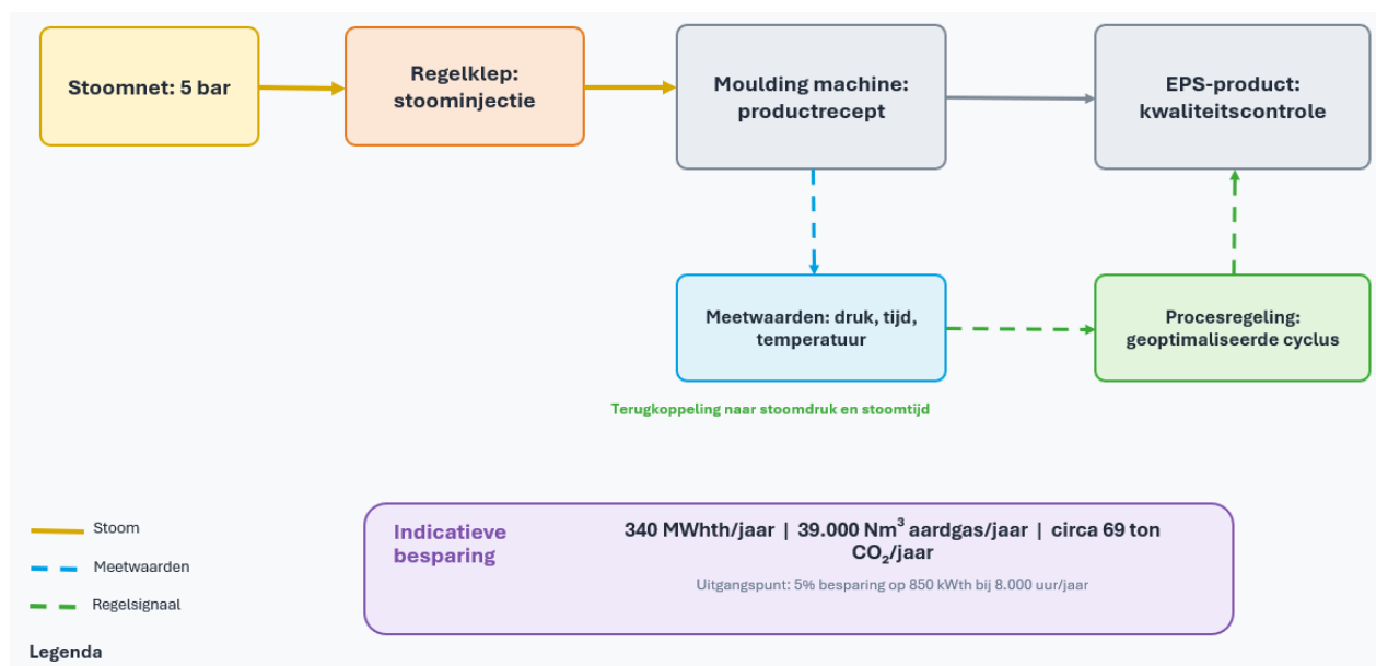
Figuur 24 – Schema maatregel 4 EPS
