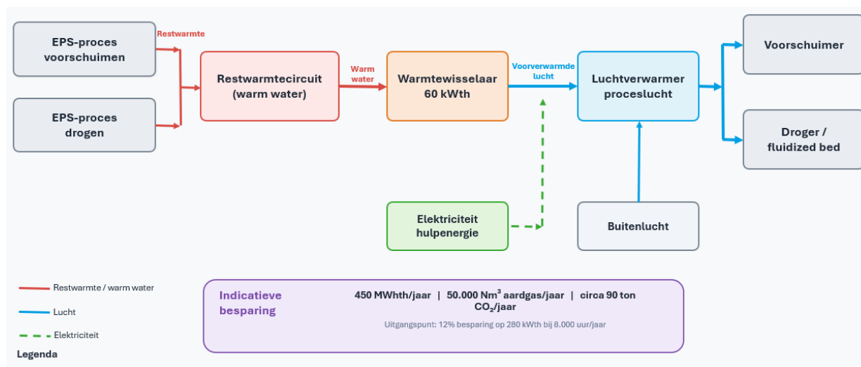
Figuur 22 – Schema maatregel 2 EPS
