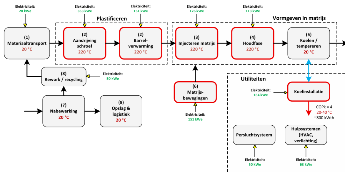
Figuur 11 – Energiebalans spuitgietproces (900 kg/h)
