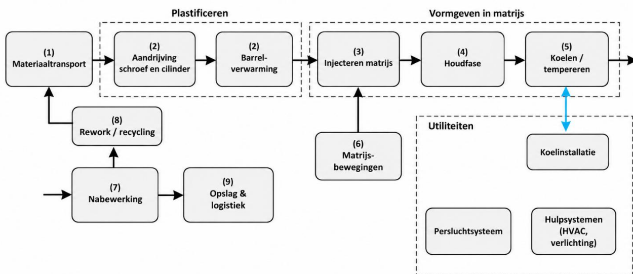
Figuur 9 – Typische spuitgietopstelling
